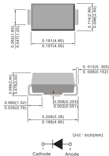
DO-214AC (SMA)
